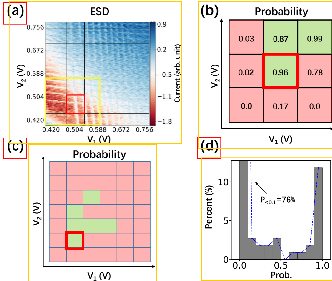
图 3.9 少电子区的搜索过程。(a) 双量子点的电荷稳定图。在处理过程中相图按照 0.06 \text{ V} \times 0.06 \text{ V} ( 31 \text{ px} ) 的大小被划分为多个部分,在此例中相图被分为 42 个部分,每一个部分将分别由 CNN 进行识别并分类。(b) CNN 给出的电荷稳定图中各区域处于双点状态的概率。图中给出了一部分详细的概率值,概率值高于 80\% 的部分被记录为双点态,低于 80\% 的部分被记录为非双点态,分别使用绿色和红色标注。(c) 完整电荷稳定图中由 CNN 给出的各区域处于双点态的概率。少电子区通过选取概率高于 80\% 的区域中拥有最低电压的部分进行定位。结果由红色框标注。(d) 相图中电荷态识别的概率分布直方图。
