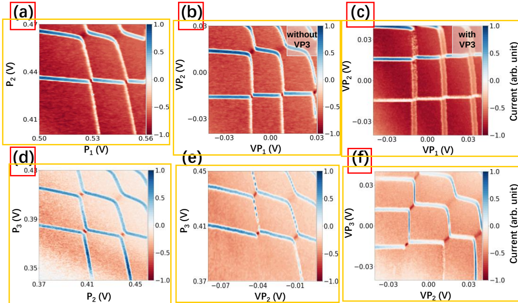
图 4.8 虚拟电极对不同量子点的影响。(a) QD_1-QD_2 的电荷稳定图。(b) VP_1-VP_2 的电荷稳定图。(c) 当加入新点 QD_3 以后重新测量的 VP_1-VP_2 电荷稳定图。可以发现少电子区的位置几乎不存在偏移。(d) QD_2-QD_3 的电荷稳定图。(e) VP_2-P_3 的电荷稳定图。在虚拟电极没有对 QD_3 进行更新之前， VP_2 和 P_2 对于 QD_3 点的影响是一样的。(f) VP_2-VP_3 的电荷稳定图。虚拟电极对 P_3 进行更新以后，抑制了 VP_2 和 VP_3 之间的串扰。
