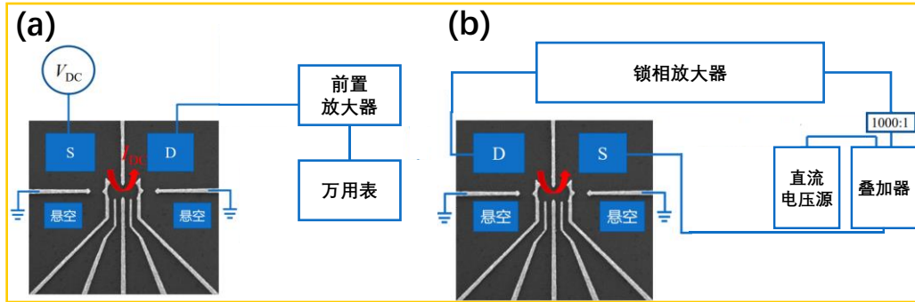
图 1.7 输运测量示意图。(a) 直流输运测量线路。(b) 交流输运测量线路。
