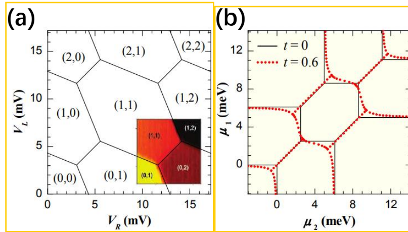
图 1.12 (a) 不考虑跃迁项的情况下计算得到的电荷稳定图。(b) 考虑跃迁项的情况下,不同隧穿耦合强度对应的电荷稳定图。(图片引自文献[48])
