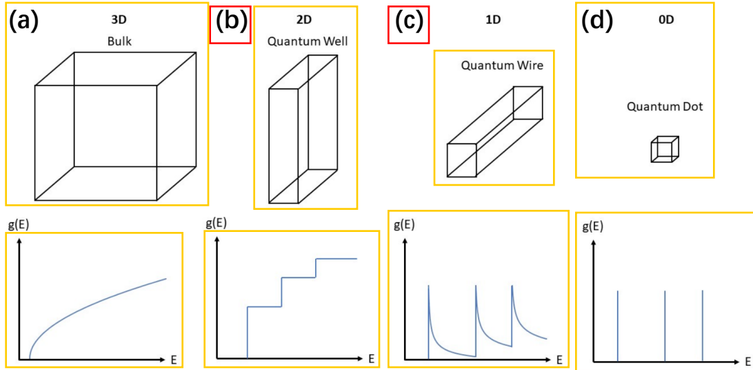
图 1.3 不同维度下能态密度的分布。(a) 三维空间中态密度是 \sqrt{E} 的函数。(b) 在二维量子阱中，态密度是一个常数，而当达到激发态能级时会产生突变。(c) 在量子线中，激发态能级位置态密度会出现奇点。(d) 在量子点中，态密度是离散分布的。
